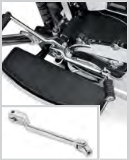
F. FOLDING HEEL SHIFTER
